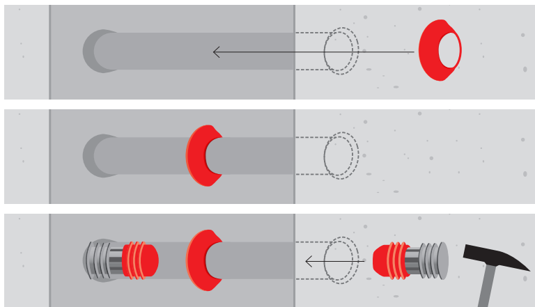
Изолация на тръба от кофражна шпилка с WEBAC® Пръстен и WEBAC® Тапа
